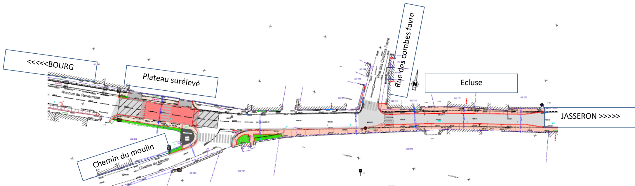
AVANT PROJET RD936 PRINCIPAUX AMENAGEMENTS ENVISAGES
